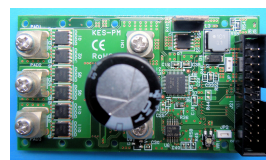
95V 100A インバータ基板
